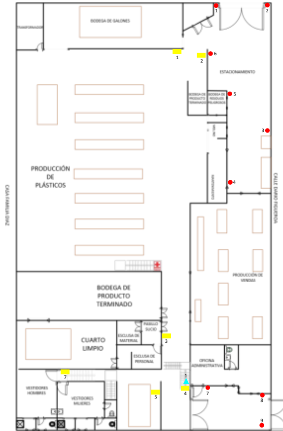
PLANTA BAJA
